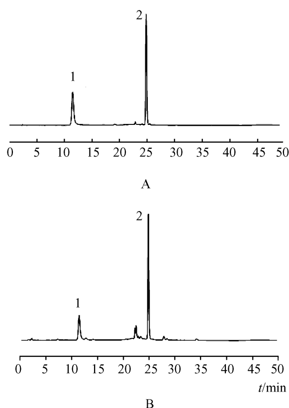
图 1 对照品 (A) 及供试品 (B) HPLC 色谱
